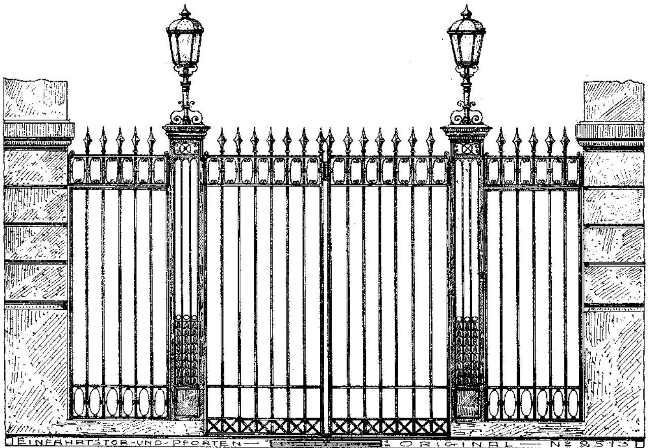
EINFAHRTSTOR - UND - PFORTEN - ORIGINAL - N° 2151 MASSSTAB
