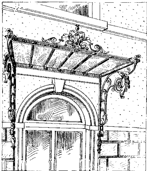
VORDACH—ORIGINAL—Nº 2642
