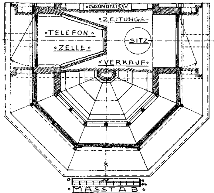
ZEITUNGS-KIOSK MIT TELEFON-ZELLE ORIGINAL-NR 2502
