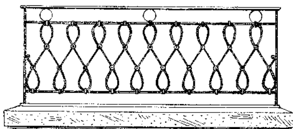
BALKONGITTER-ORIGINAL-Nº 2756
